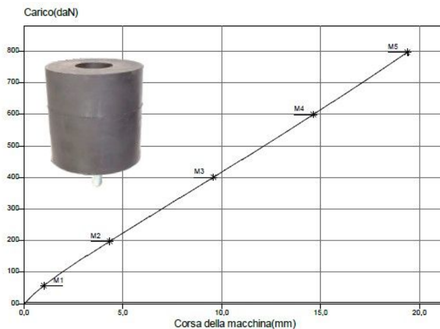
TEST CARICO/CEDIMENTI a compressione assiale per durezza sh.67
